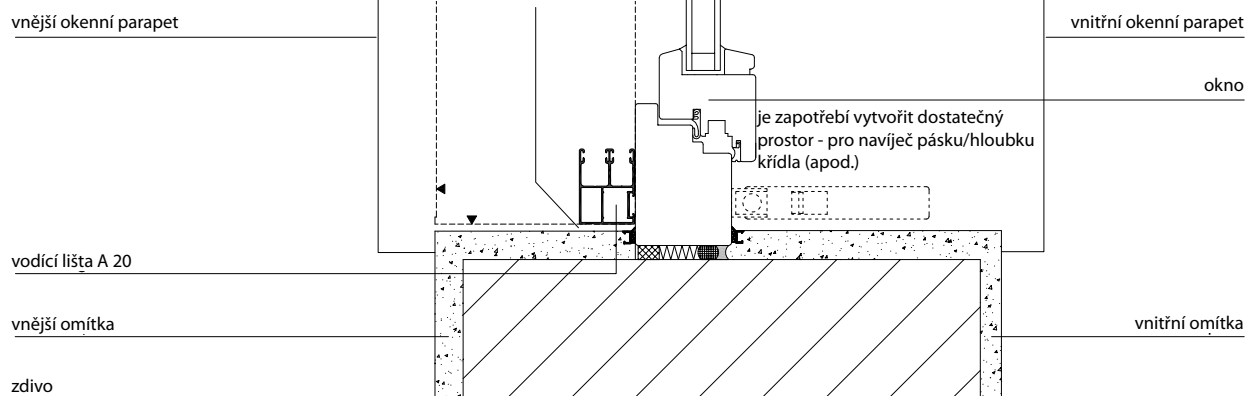
detail spojení - pohled z boku (dolní část)
